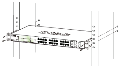
圖 3. 安裝交換器到標準尺寸的機架
