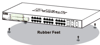
Рисунок 1. Крепление резиновых ножек
