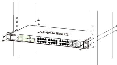
Gambar 3. Memasang switch ke rak dengan ukuran standar
