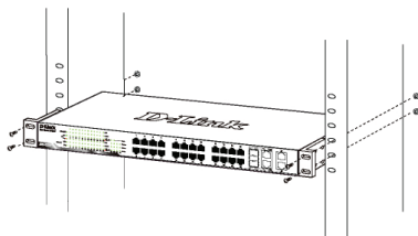
Figura 3. Instalar el switch en un rack estándar
