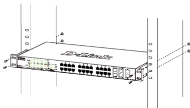
图3. 安装交换机到标准尺寸的机架
