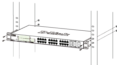
Abbildung 3: Switch im Standardrack installieren
