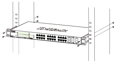
Figura 3. Instalando o switch em um rack de equipamentos tamanho padrão
