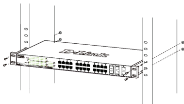
図3 スイッチをラックに取り付ける
