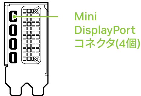
RTX 4000 SFF
